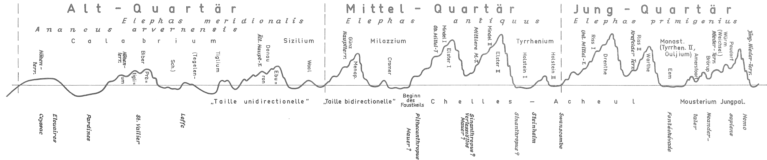
Tafel 1. Schematische Kurve, den Ablauf des Eiszeitalters verdeutlichend, hauptsächlich für Mitteleuropa gültig.
