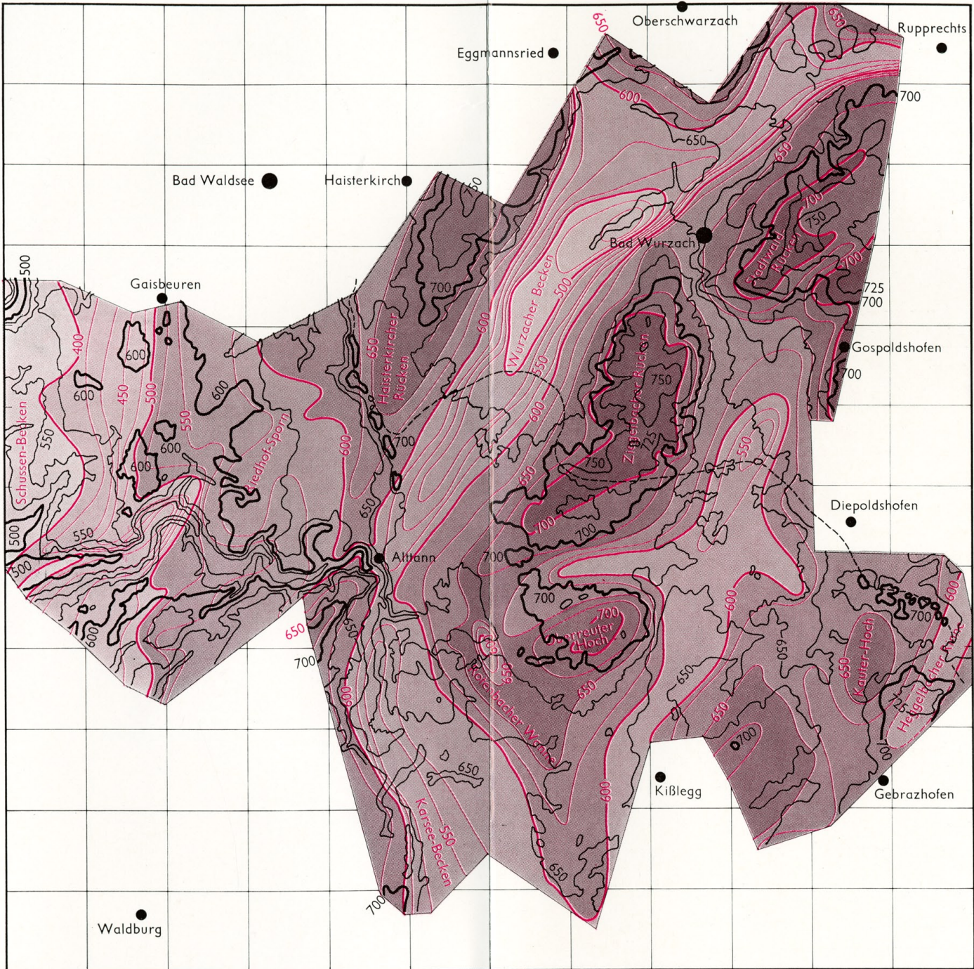
Höhenlage der Tertiär/Quartär-Grenze im mittleren Oberschwaben (rot) und der heutigen Erdoberfläche (schwarz).
