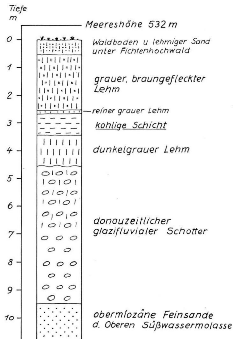
Abb. 2. Stratigraphisches Profil des Uhlenberg-Interglazials.
