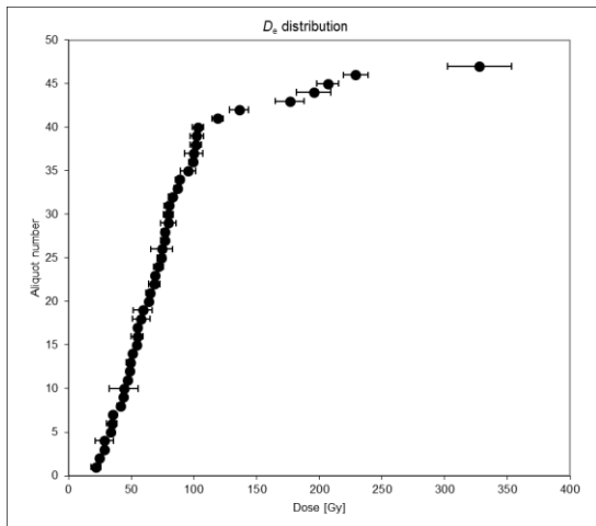
SZB-1 feldspar IR50 (1 mm aliquots)
