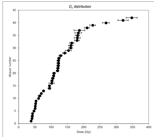
SZB-2 feldspar IR50 (1 mm aliquots)
